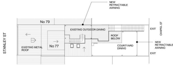
1 SITE PLAN/ROOF PLAN 1 : 200
