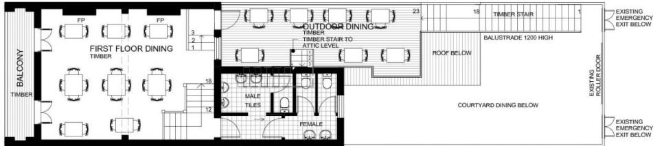
2 EXISTING LEVEL 1 1 : 100
